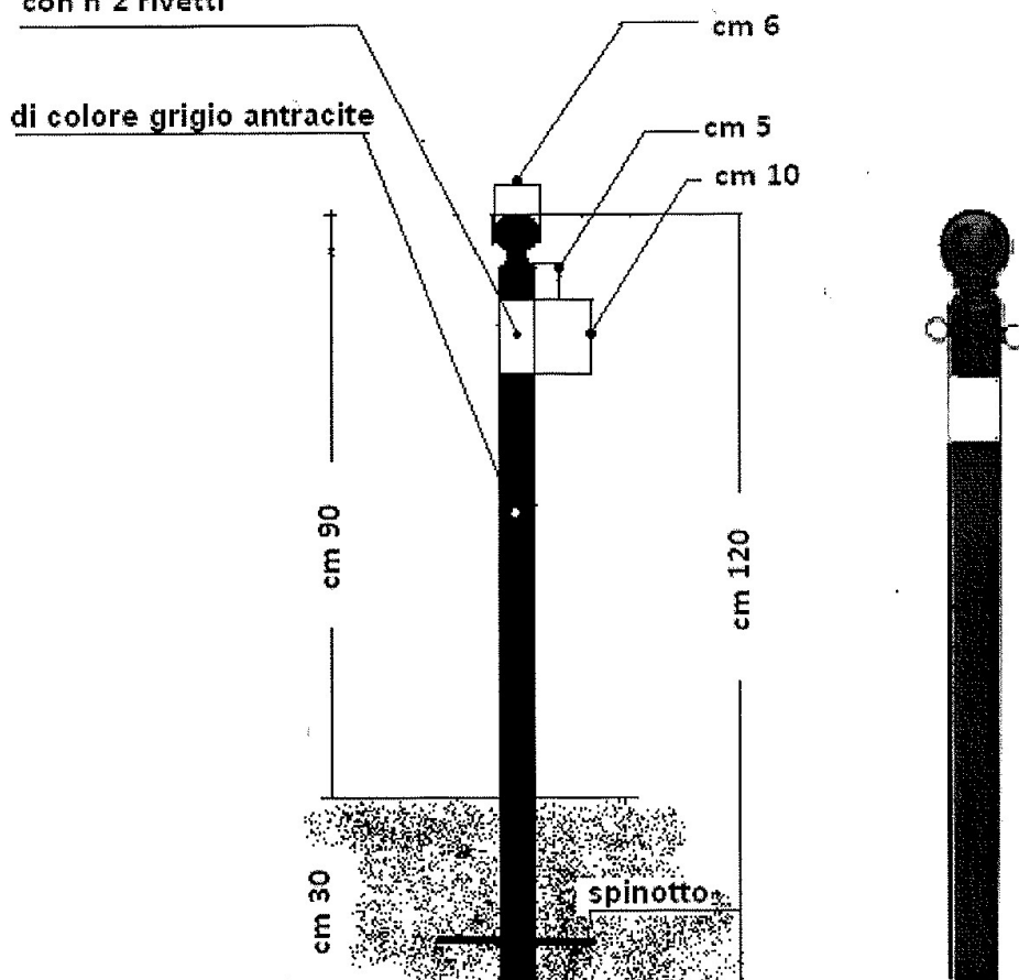
DISSUASORE PALETTO PARAPEDONALE TUBOLARE CIRCOLARE
